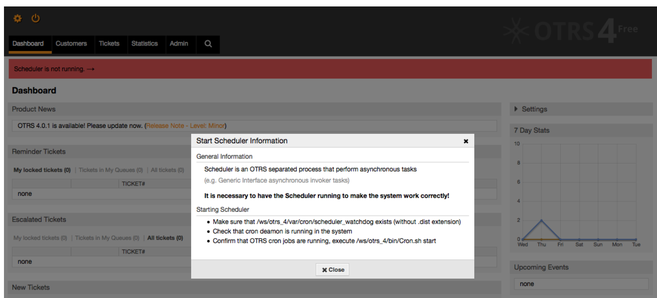
Рисунок: Запуск Планировщика.
