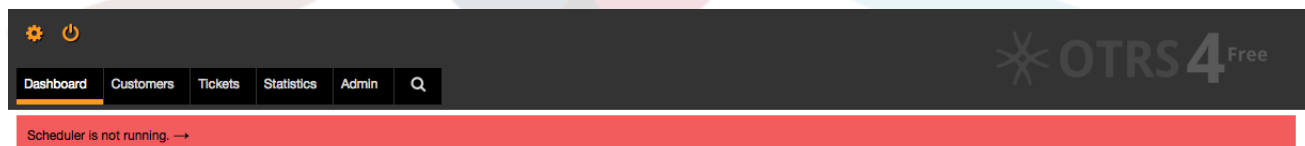
Figure: Уведомления планировщика.
