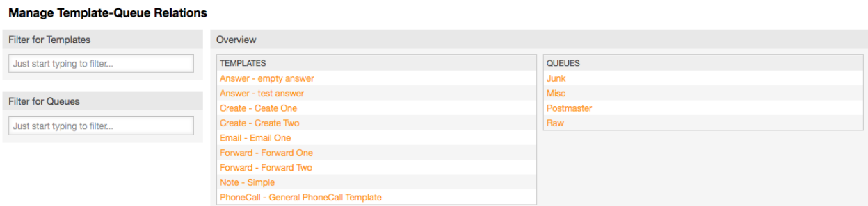
Рисунок: Управление связями Шаблон - Очередь.
