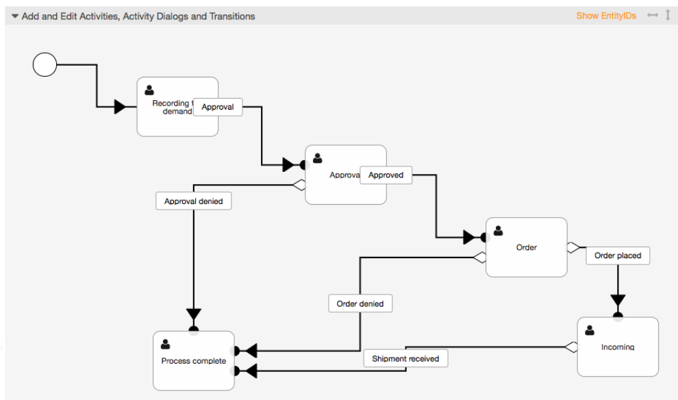
Рисунок: Полная схема процесса заказа книги.
