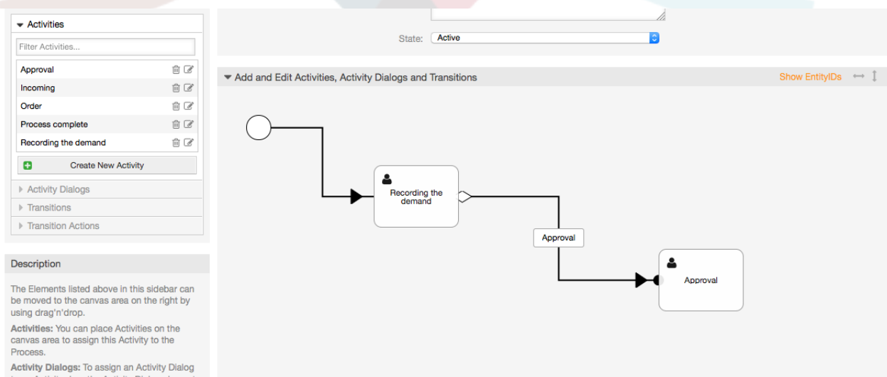
Рисунок: Связать Активности используя Переходы.
