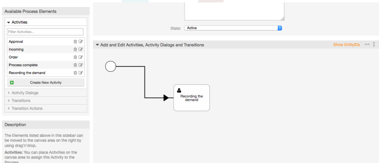
Рисунок: Помещение первой Активности на полотно схемы.
