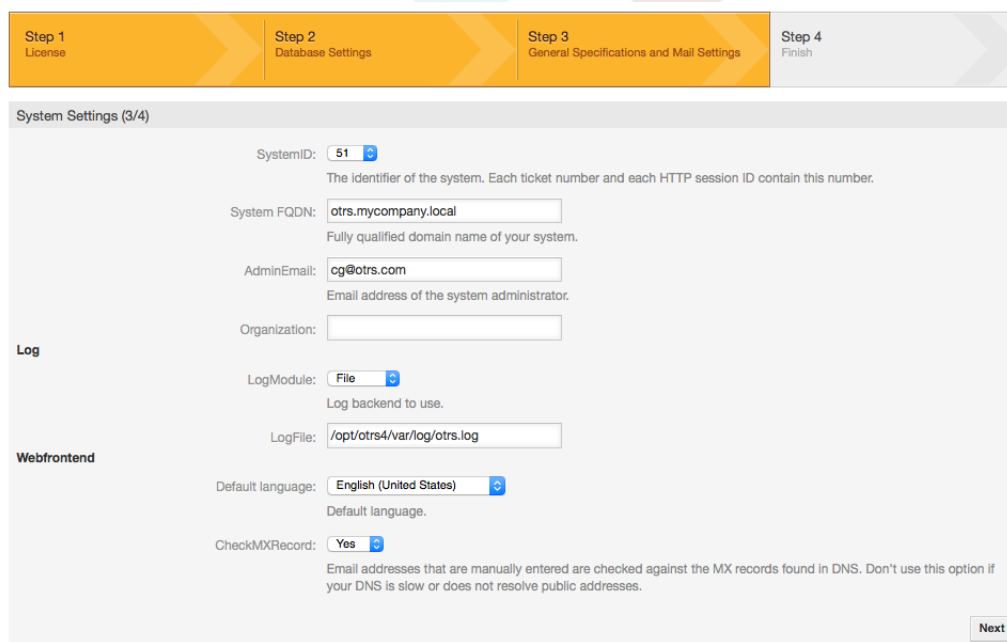
Рисунок: Настройки системы.
