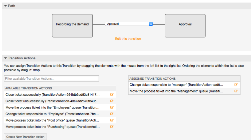
Рисунок: Назначение Действий Перехода.
